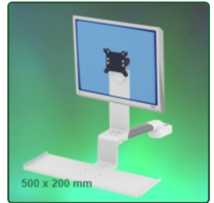
Bras Médical Standard Combo Horizontal de 240 mm Montage sur Pole Fixe 25 mm
