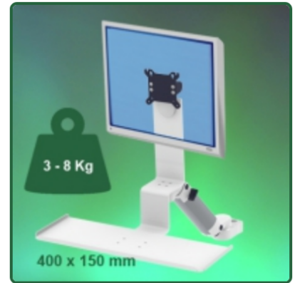
Bras Médical Standard Combo Ajustable en hauteur de 300 mm Montage sur Pole Fixe 25 mm Référence: 998.105-2-2
