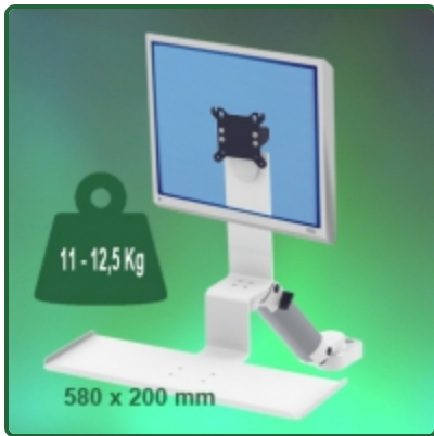
Bras Médical Standard Combo Ajustable en hauteur de 300 mm Montage sur Pole Fixe 25 mm
