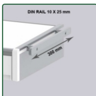
Din Rail 10 x 25 mm. Length 300 mm.
