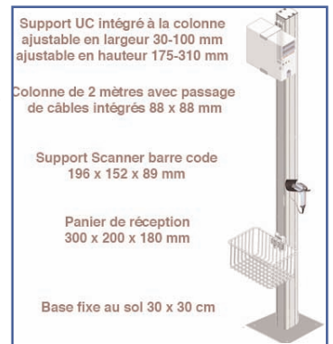
Fixation Colonne
