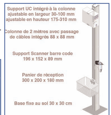
Fixation Colonne
