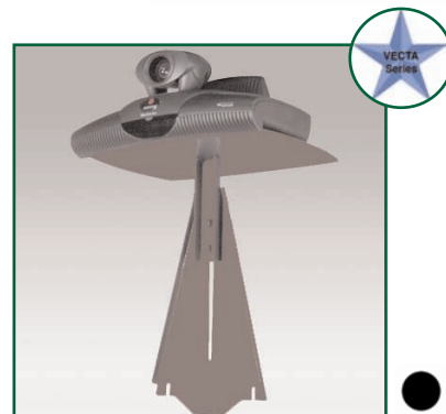
Référence: EGF 78AVCMB Support Vidéo Conférence Vecta Serie Matériaux: Aluminium Dimensions: 26 x 34 cm Poids supporté: 3 KG
